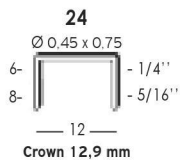
Crown 12,9 mm
