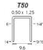
Crown 9,9mm
