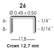
Crown 12,7 mm
