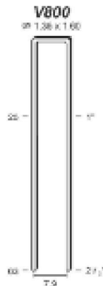
Crown 7,9mm
